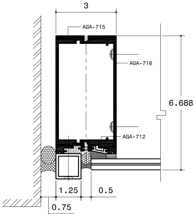
JAMB DETAIL
